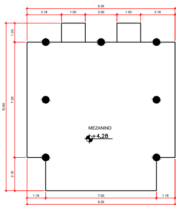
PLANTA — MEZANINO
