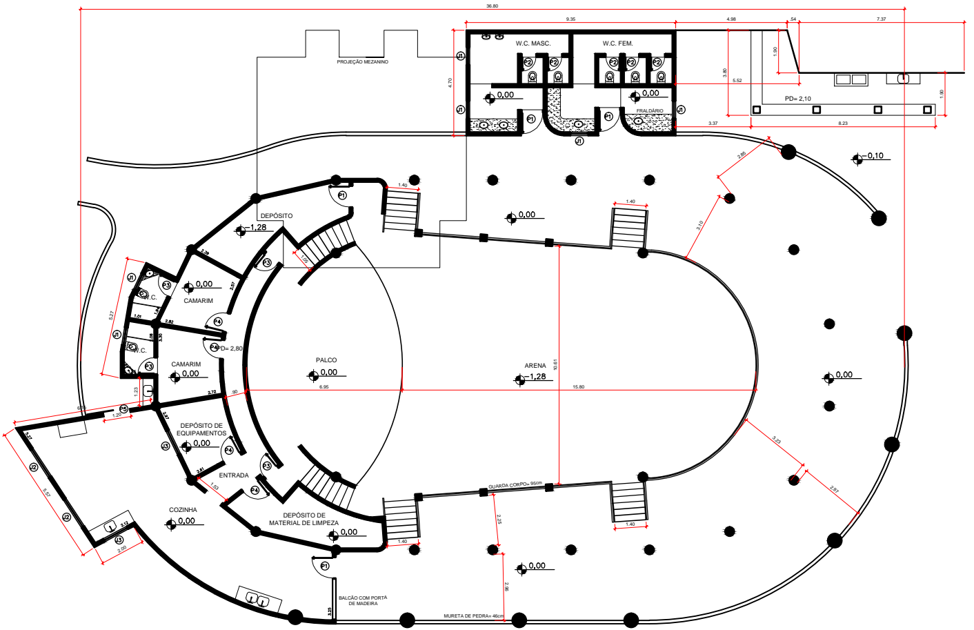
PLANTA — ARENA
